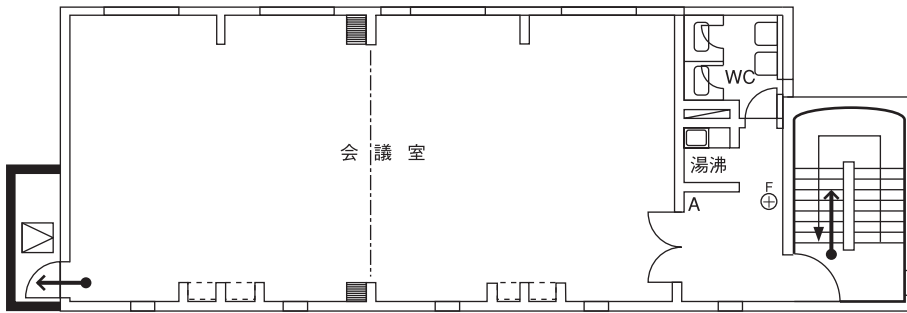
2階平面図
